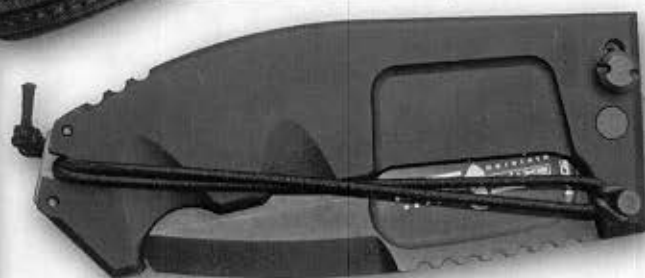
Le pliant RAO fermé avec la goupille de sécurité en position. Il est impossible de faire pivoter la lame.
